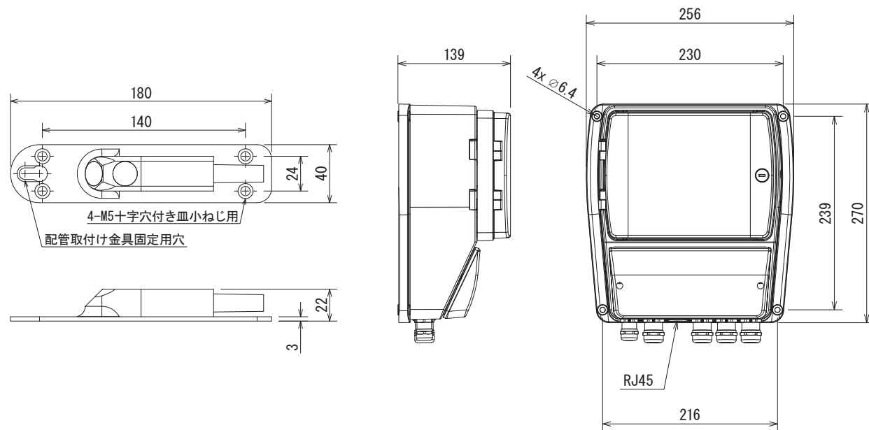
流速・水位複合センサー CSW-10型
