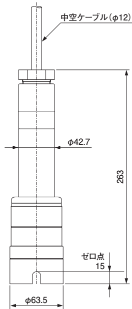
SL-710C型
