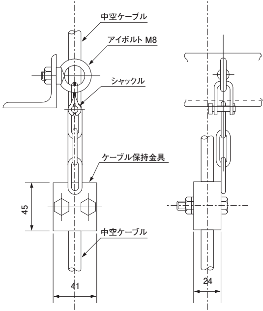
中空ケーブル保持金具 (薬液槽は除く)
