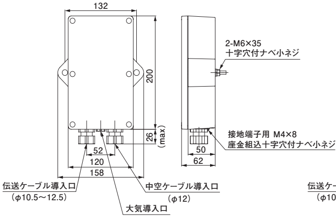
JB-56□S型
