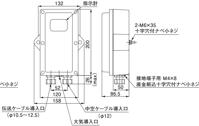
JB-56□M型
