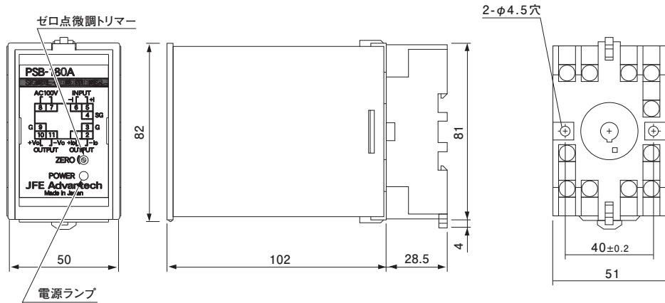
PSB-180□,182□型
